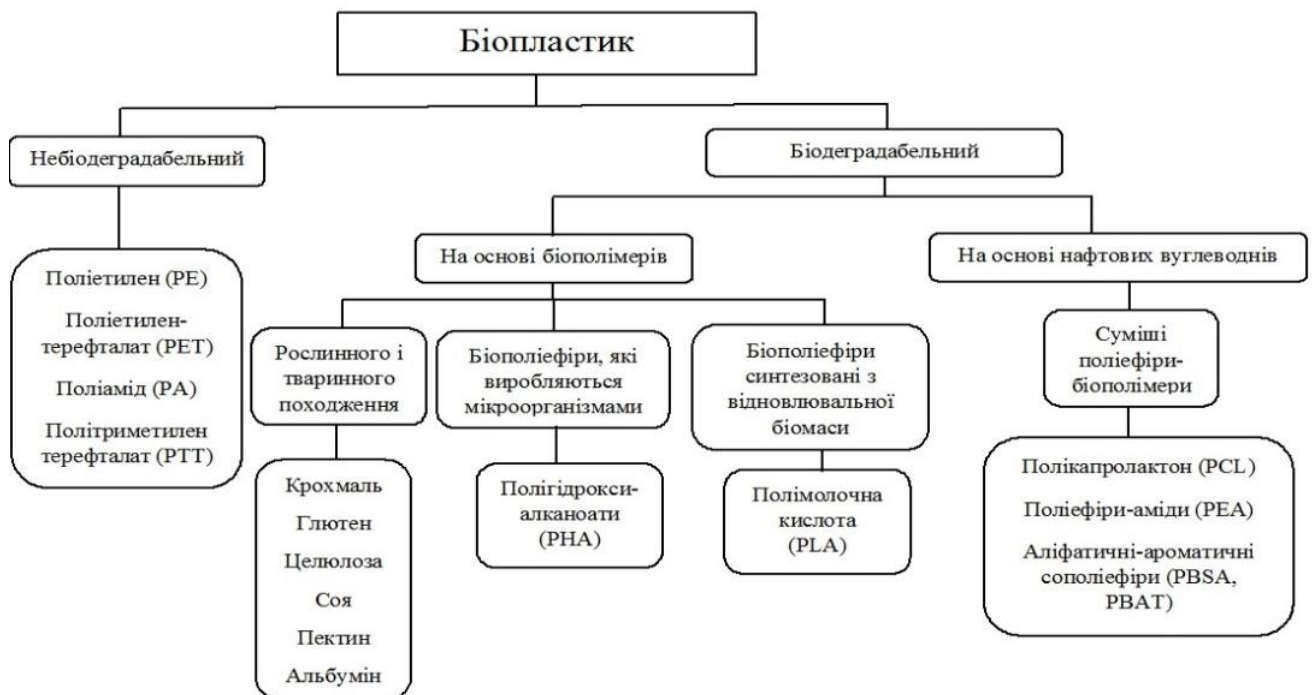
Рис. 2.1. Види біопластику [1]
